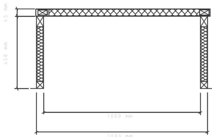
Skiss över uppstigningslucka, VULi1010
